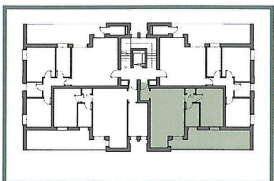
UBICAZIONE AL PIANO Piano Terzo
